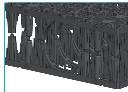
Steg 6: "Klicka" ihop dem.
