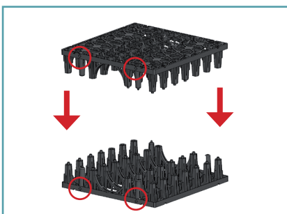
Steg 4: Säkra att pilarna på halvorna pekar mot varandra.
